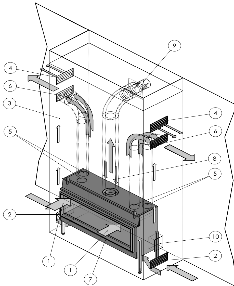
Figuur 16: Toestel ingebouwd in geventileerde schouw Horizontale uitmondung van de rookgasafvoer/verbrandingslucht- toevoer via de muur.
