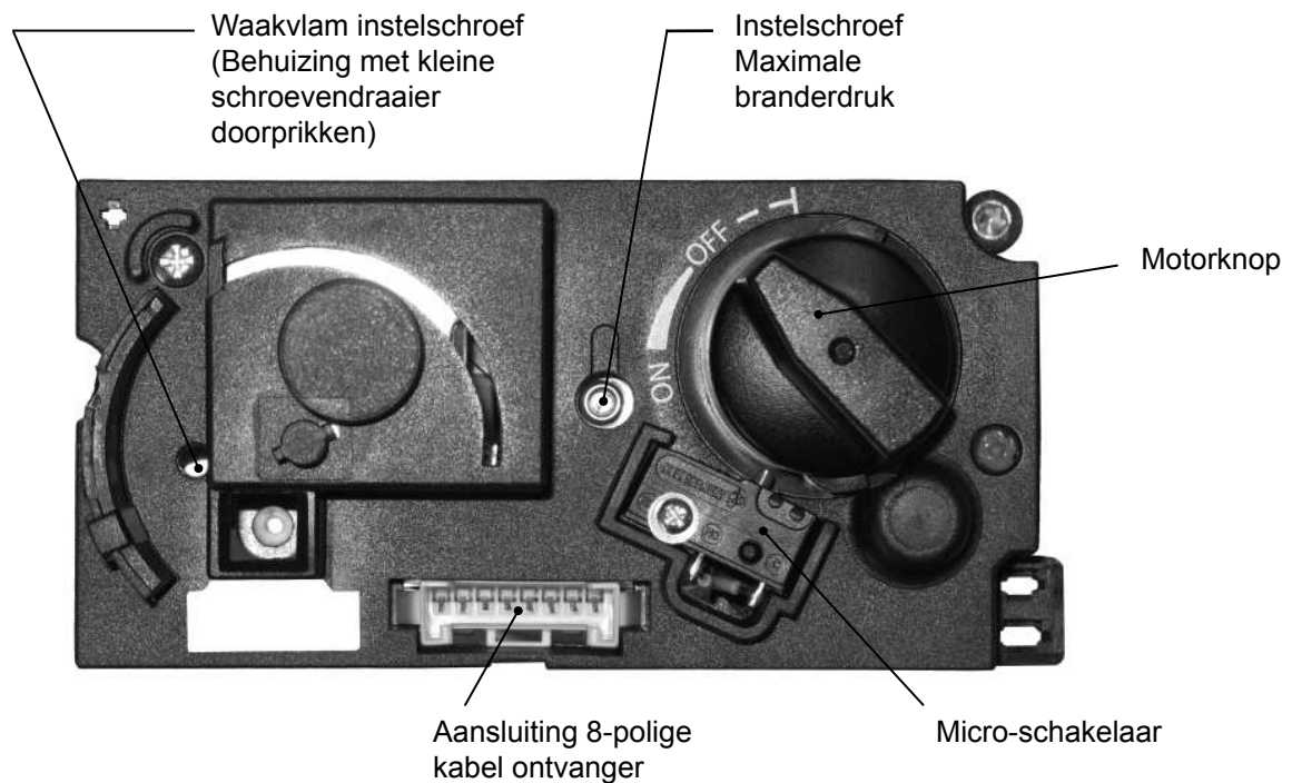
Figuur 20: Gasregelblok - Voorzijde
