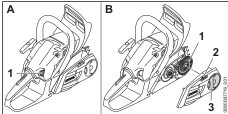
Kraftstoffhandpumpe (A)
