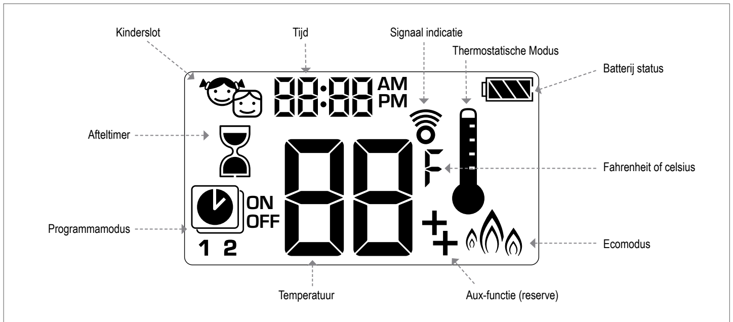
Afb. 21: 8-symbool Display
