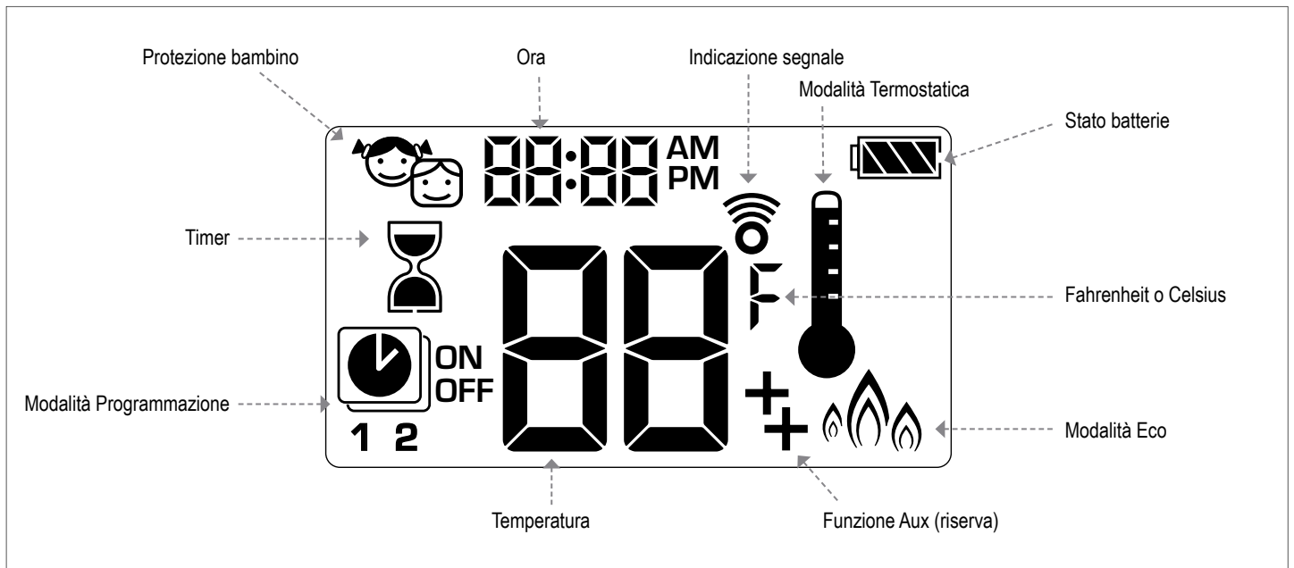
Fig. 21: Display a 8 caratteri
