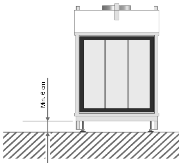
Figuur 15: Minimaal 6 cm ruimte tussen onderzijde toestel en vloer
