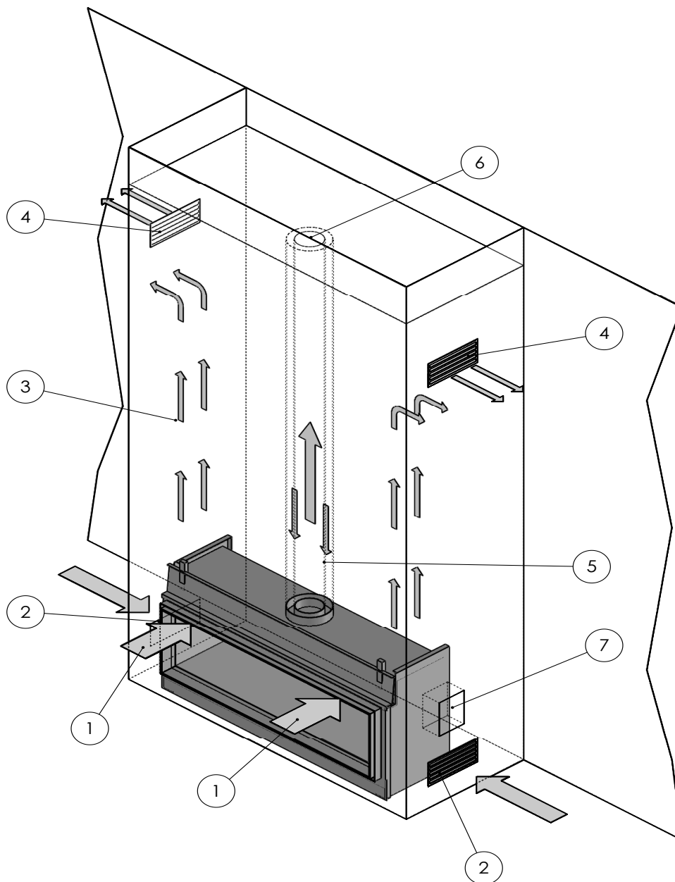
Figuur 17: Toestel ingebouwd in geventileerde schouw Verticale uitmondung van de rookgasafvoer/verbrandingslucht- toevoer via het dak. Toepassing zonder convectiepakket
