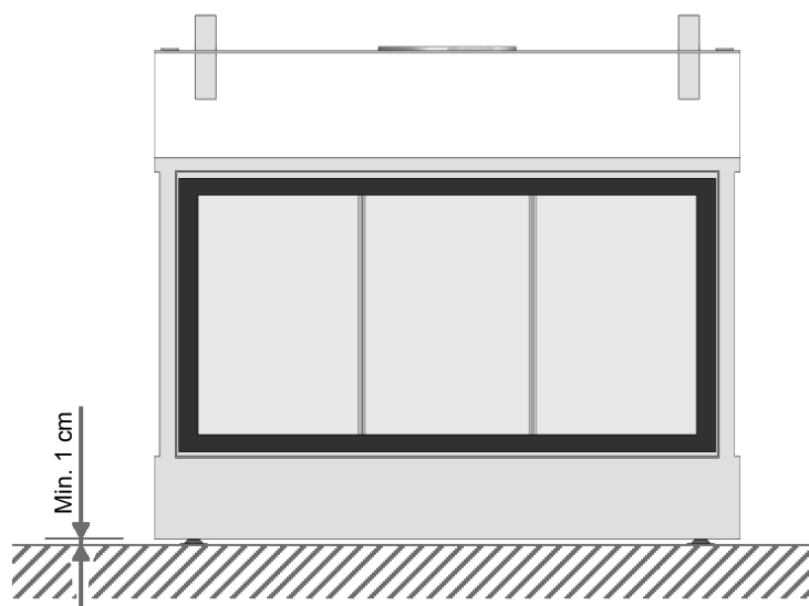
Figuur 15: Minimaal 1 cm ruimte tussen onderzijde toestel en vloer
