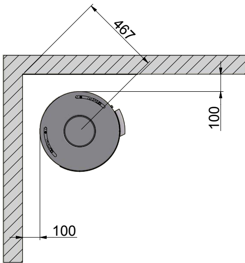
45° hoekopstelling
