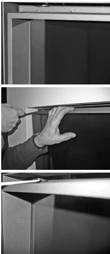
- Trek met de haak, middenboven, de dunne, metalen veer-strip van het nokje van het frame af.
