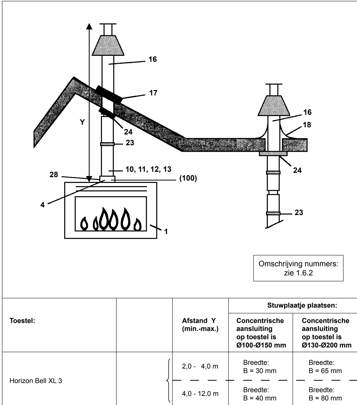
Figuur 4: Verticale dakuitmondung zonder versleping
